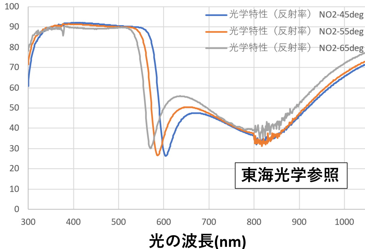
コールドミラーの反射スペクトル No2
